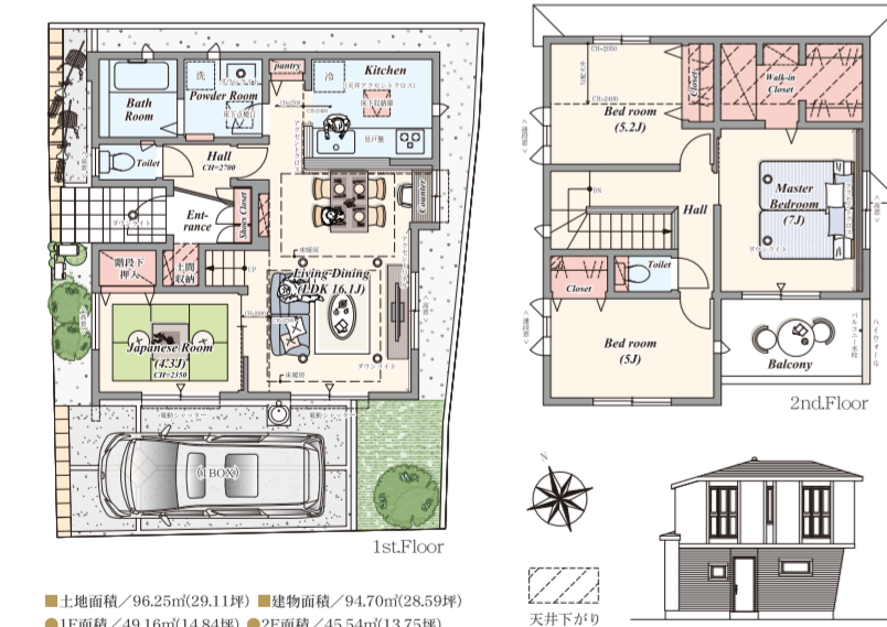
※掲載の間取りは計画図より作成の為、詳細に関しては設計図書・外構図面にてご確認ください。※各区分画図は計画図の図面を基に描き起こしたもので、実際とは異なります。
